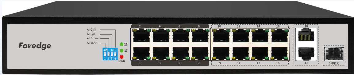
الواجهة الأمامية – 16 منفذ PoE ومنفذ رابط جيجابت ومنفذ SFP combo ووزر الأوضاع الذكية
