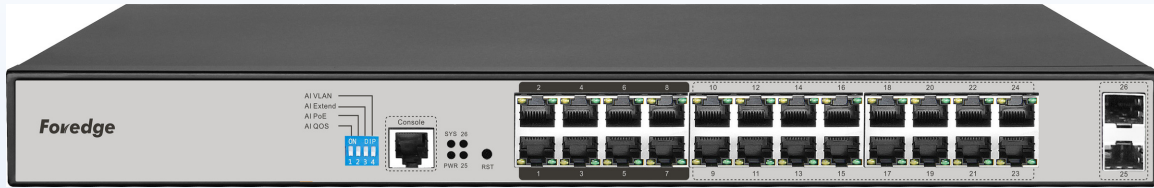
الواجهة الأمامية – 24 منفذ PoE جيجابت ومنفذ ألياف SFP ومنفذ كونسول وزر الأوضاع الذكية
